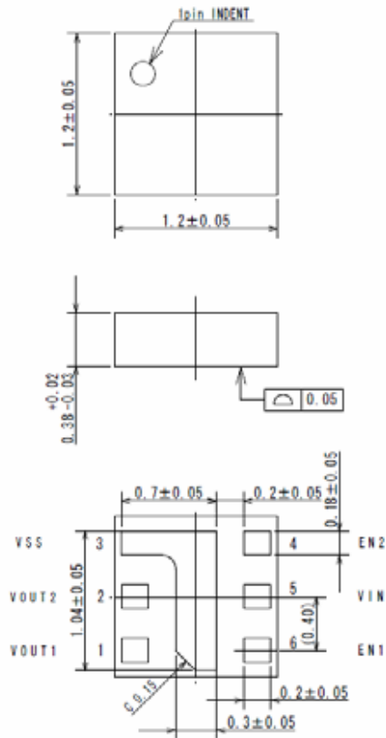
USP-6B04
