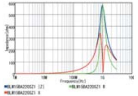
BLM15BA220SZ1
