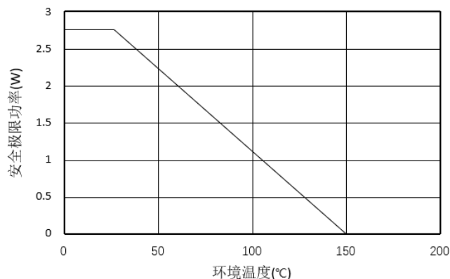
图 6.热降额曲线, 依据 DIN V VDE V 0884-11 的安全限值与环境温度的关系(左: π14xU3x; 右: π14xU6x)
