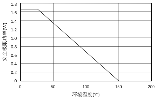
图 6.热降额曲线, 依据 DIN V VDE V 0884-11 的安全限值与环境温度的关系(左: π14xU3x; 右: π14xU6x)
