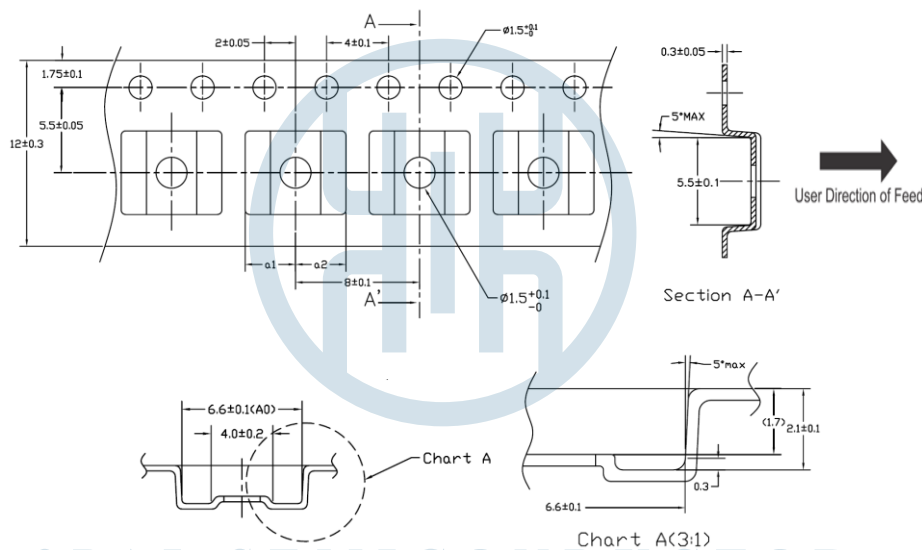
图 27. 16 引脚宽体 SSOP 封装包装信息-尺寸单位(mm)
