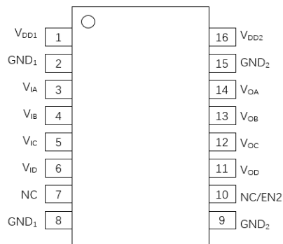
图 3.π140Uxx 管脚定义
