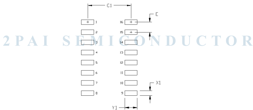
图 21. 16 引脚窄体 SOIC 封装 [NB SOIC-16] 焊盘图案
