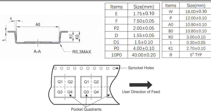
图 26. 16 引脚宽体 SOIC 封装 [WB SOIC-16] 包装信息
