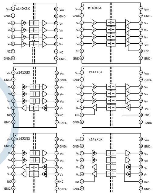
图 1. \pi 140xxx/ \pi 141xxx/ \pi 142xxx 功能框图
