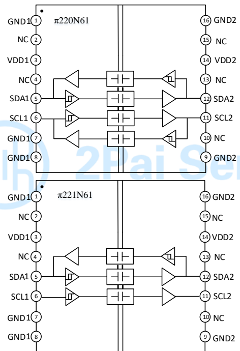
图 1. π220N61/π221N61 功能结构框图
