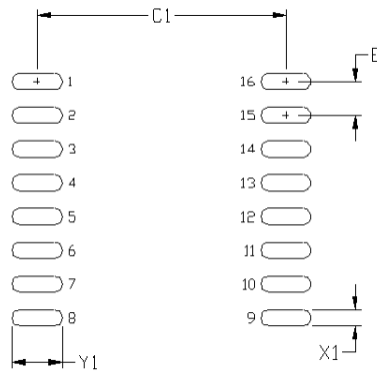
图 24.8 引脚标准小型封装窄体 SOIC-8
