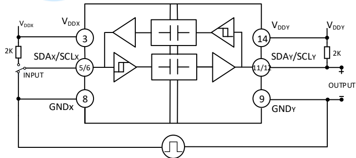
图 19. 共模瞬变抗扰度测试电路图
