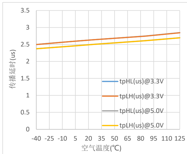
图 8.π13xU6x 传输延时 vs. 空气温度
