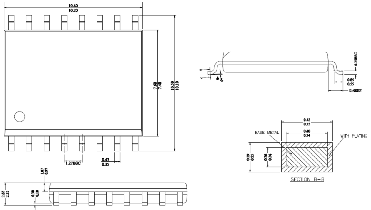
图 14. WB SOIC-16 封装外形尺寸-尺寸单位(mm)
