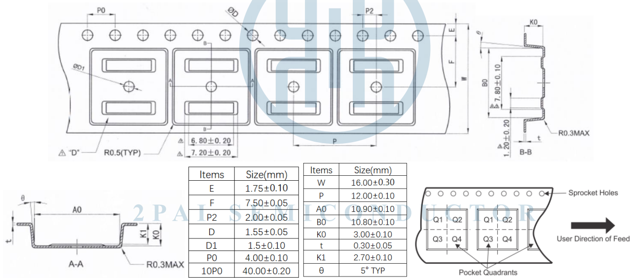
图 45.WB SOIC-14 包装示意图
