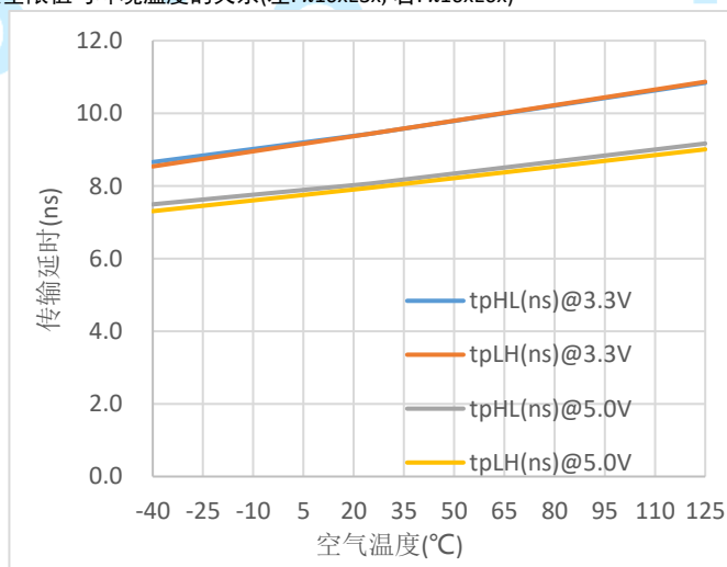
图 9.π16xE3x 传输延时 vs. 空气温度
