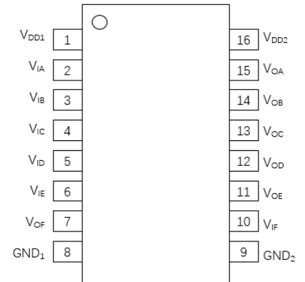
图 4. \pi 161Exx 管脚定义
