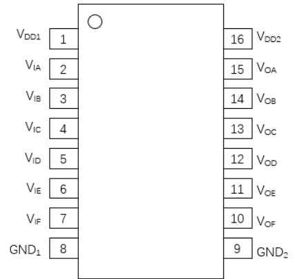
图 3. \pi 160Exx 管脚定义
