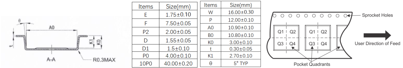
图 22.16 引脚宽体 SOIC 封装 [WB SOIC-16] 包装信息
