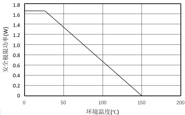
图 7.热降额曲线, 依据 DIN V VDE V 0884-11 的安全限值与环境温度的关系(左: π16xE3x; 右: π16xE6x)
