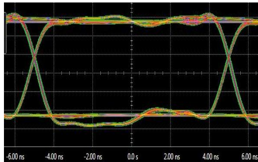
图 14. \pi 16XExx 眼图
