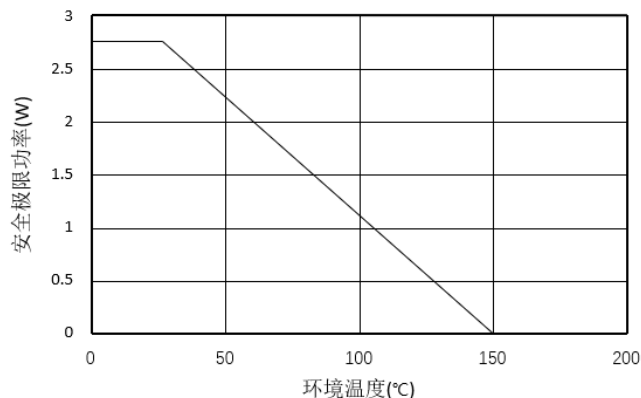
图 7.热降额曲线, 依据 DIN V VDE V 0884-11 的安全限值与环境温度的关系(左: π16xE3x; 右: π16xE6x)
