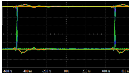
图 13. \pi 14xMxx 眼图
