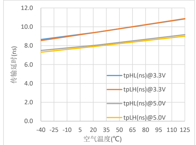
图 8.π14xM3x 传输延时 vs. 空气温度
