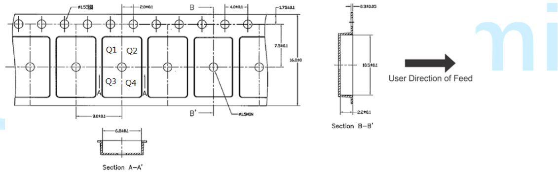
图 22. 16 引脚窄体 SOIC 封装 [NB SOIC-16] 包装信息-尺寸单位(mm)
