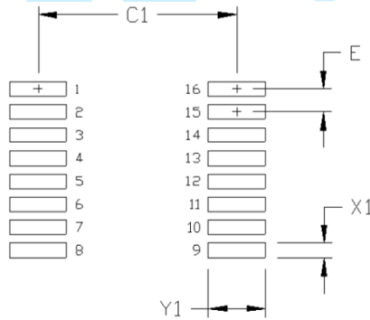
图 20. 16 引脚 SSOIC 封装 [16-Lead SSOP] 焊盘图案
