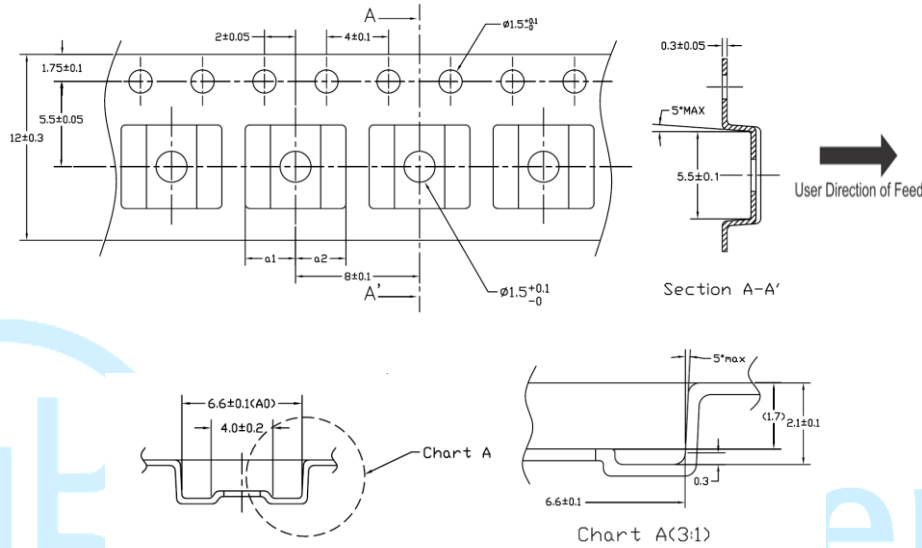
图 24. 16 引脚宽体 SSOP 封装包装信息-尺寸单位(mm)
