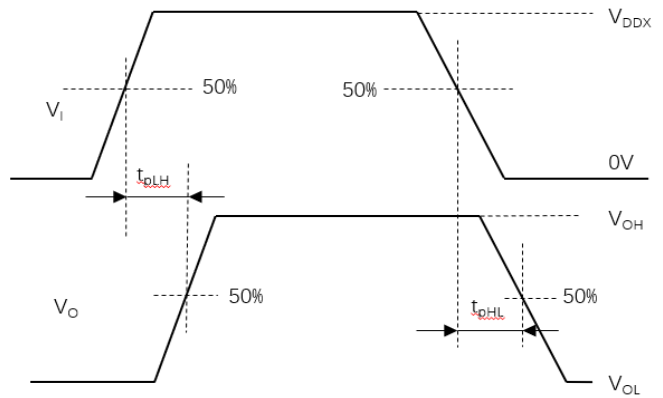
图 11. 传输延迟时间波形测量
