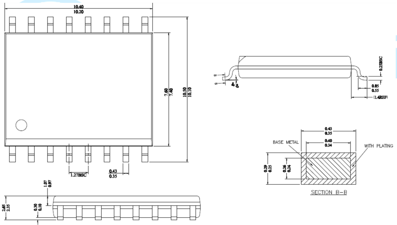
图 16. WB SOIC-16 封装外形尺寸-尺寸单位(mm)
