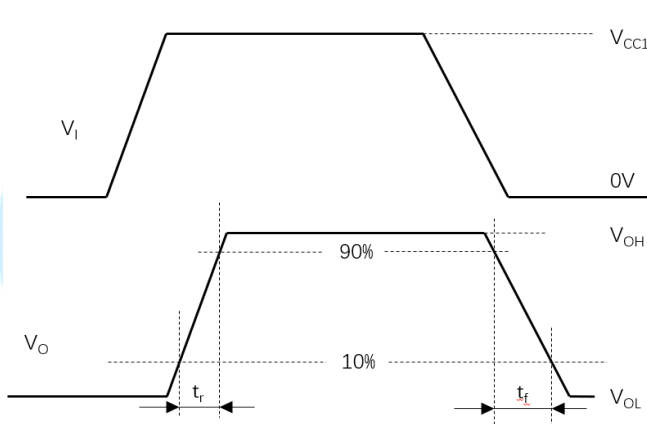
图 10. 传输时间波形测量
