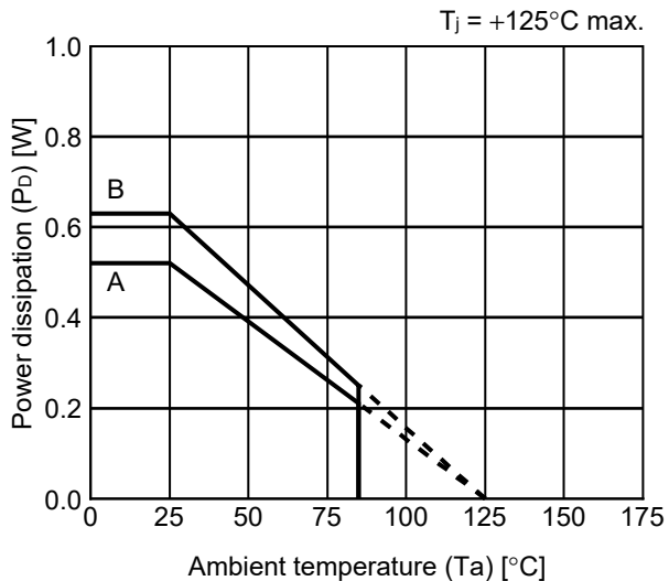
SOT-23-5
