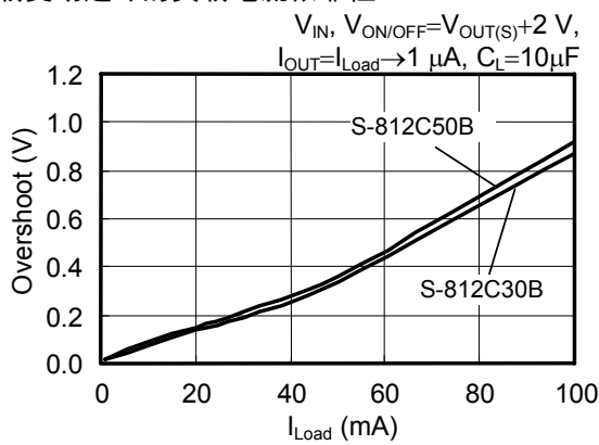
负载变动过冲的负载电流依赖性
