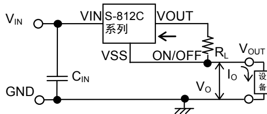
图 19 定电流电路
