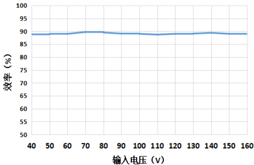
效率VS输入电压 (满载)
