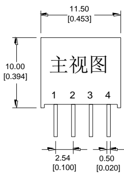
封装尺寸图
