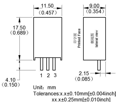
封装尺寸图
