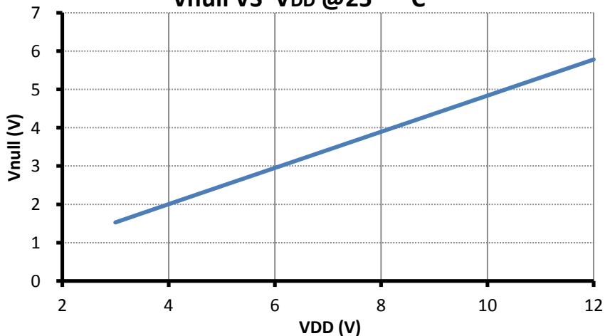
Vnull VS VDD @25 ° C
