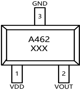
SOT23
