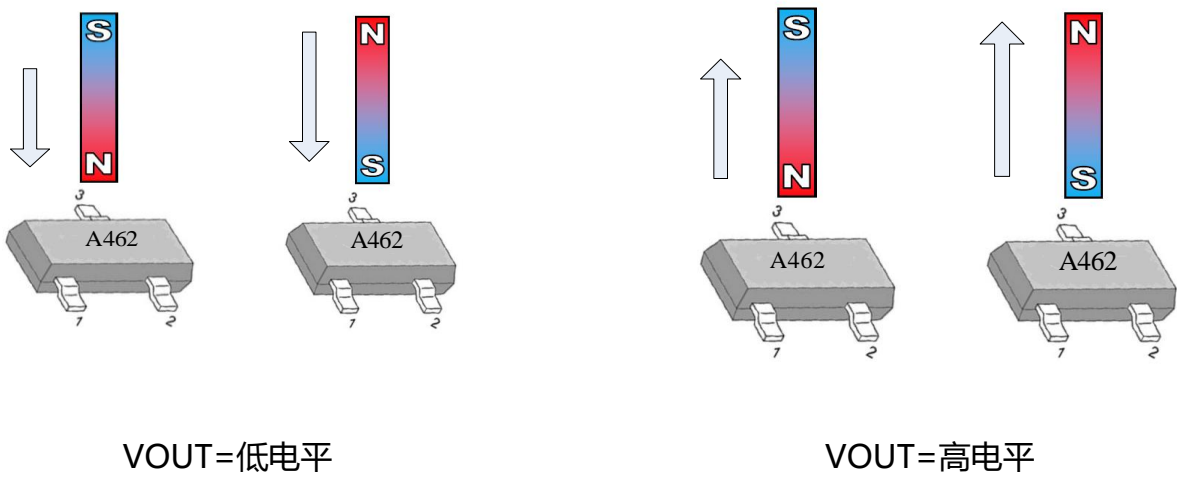
SOT23 (AH462SU)
