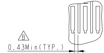
Detail: F
