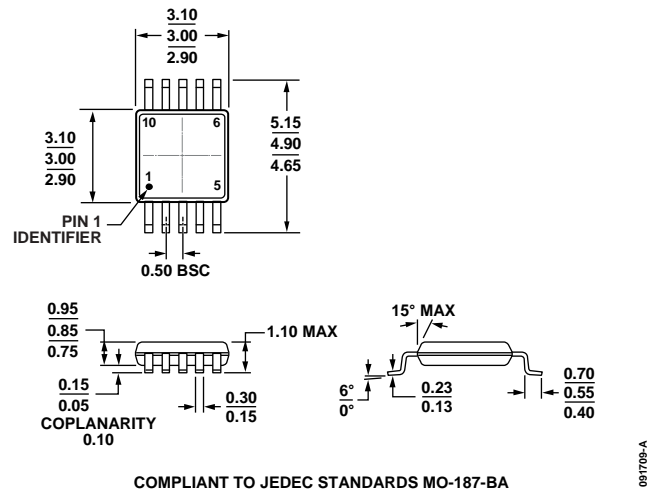
图49. 10引脚超小型封装[MSOP] (RM-10) 图示尺寸单位: mm
