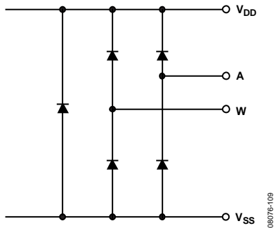
图48. 由 V_{DD} 和 V_{SS} 设置的最大端电压
