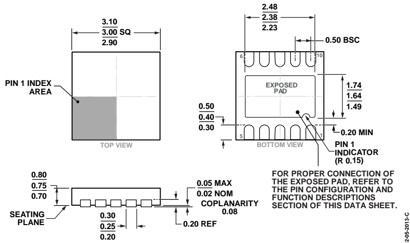
图50. 10引脚框架芯片级封装[LFCSP_WD] 3 mm x 3mm, 超薄体, 双引线 (CP-10-9) 图示尺寸单位: mm
