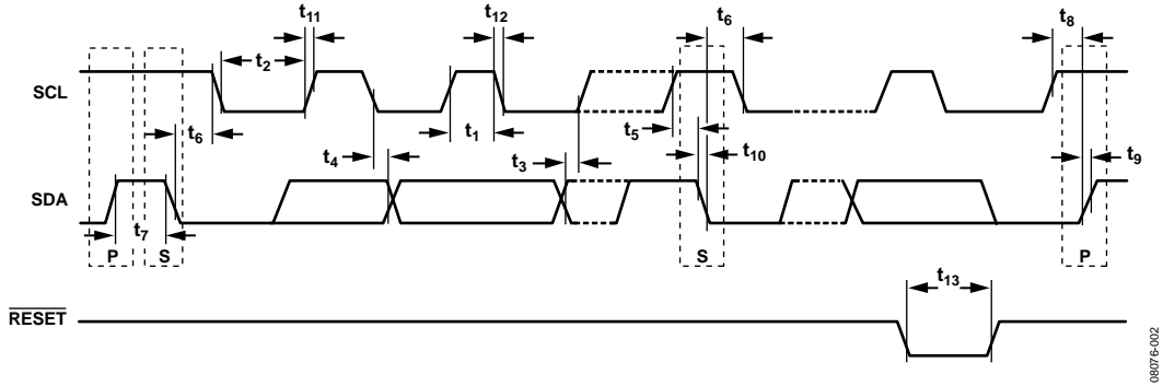
图3. 双线式串行接口时序图
