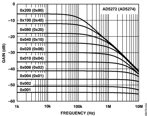
图26. 50 kΩ增益与代码和频率的关系
