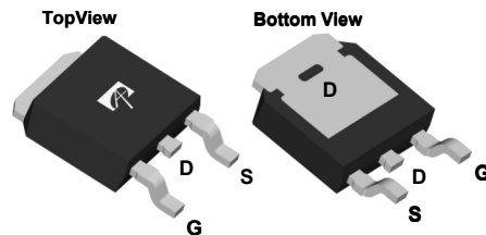
TO252 (DPAK)
