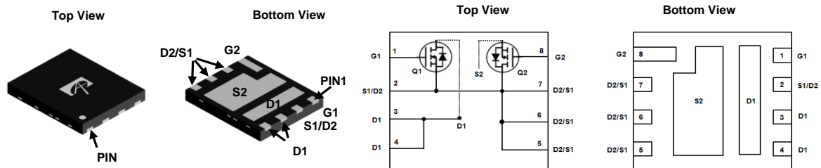
DFN 5X6E
