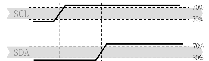
图 11 停止传输状态 (P) - 当 SCL 高电平时，SDA 线上从低电平转换为高电平。停止状态是由主机控制的一种特殊的总线状态，指示从机传输结束（Stop 之后，BUS 总线一般被认为处于闲置状态）。
