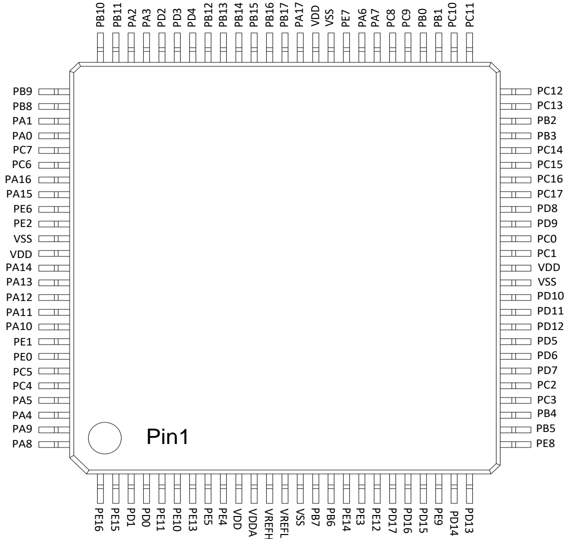
图 9-2 LQFP100 封装
