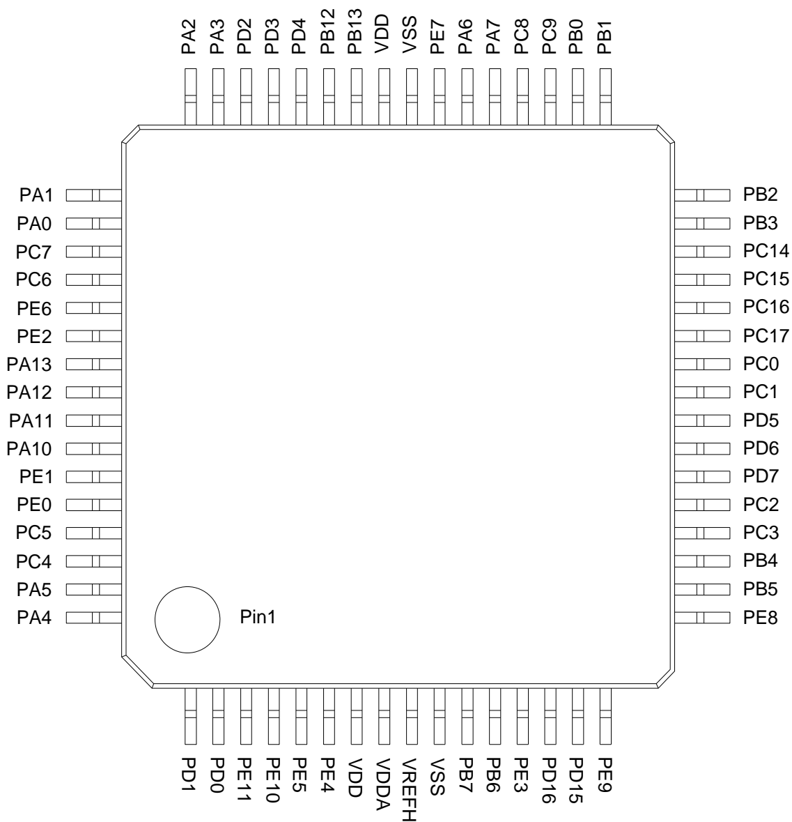
图 9-3 LQFP64 封装
