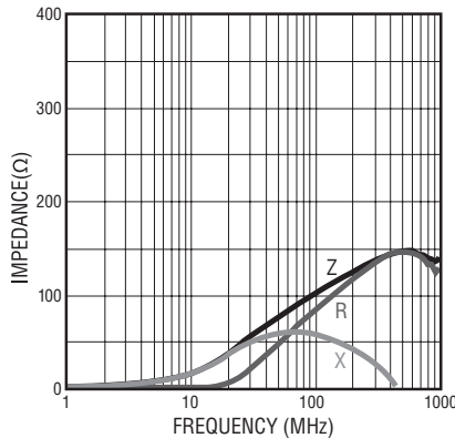
MH 1608- 101Y
