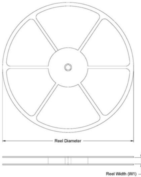
REEL DIMENSIONS
