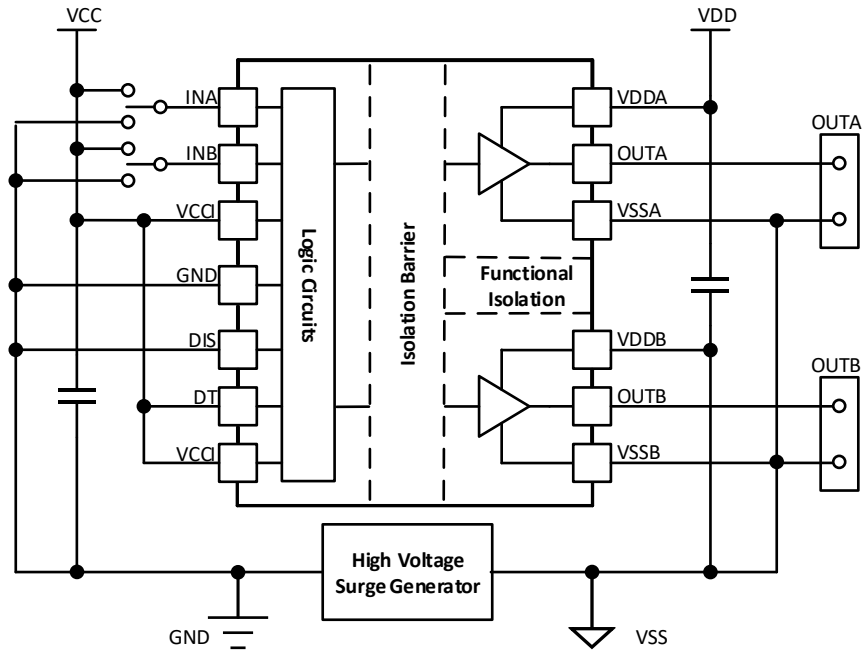
图 8-6. 共模瞬态抑制(CMTI)测试电路
