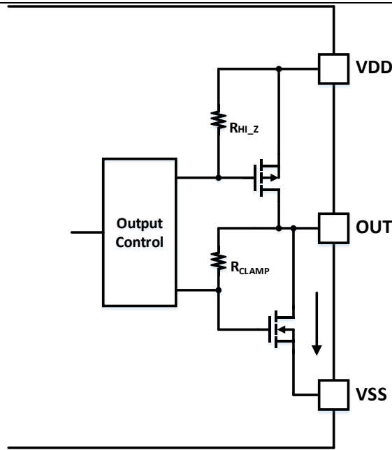
图 9-3. 有源下拉
