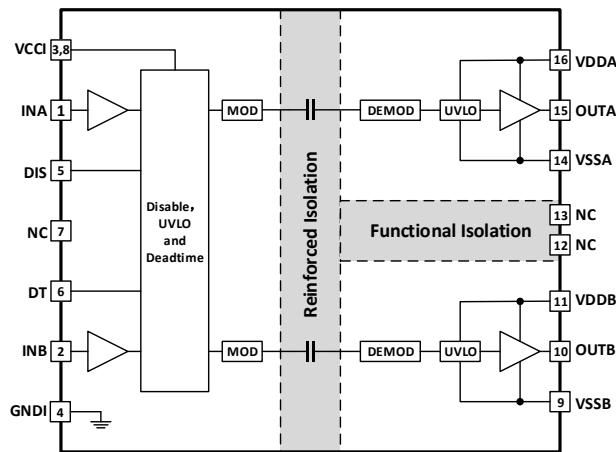
简化框图
