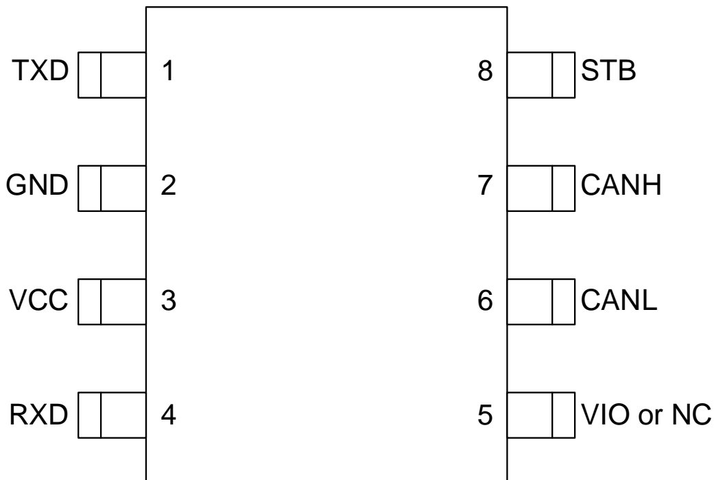
图 5-1 CA-IF1044-Q1 引脚图
