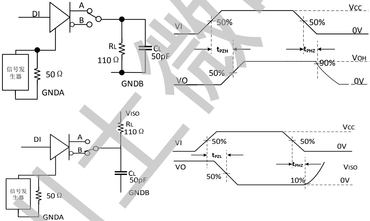
图 10-8 驱动开启和关闭时间
