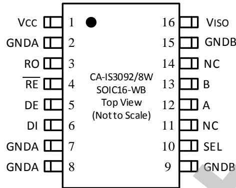
图 6-1 CA-IS3092W/CA-IS3098W SOIC16 配置
