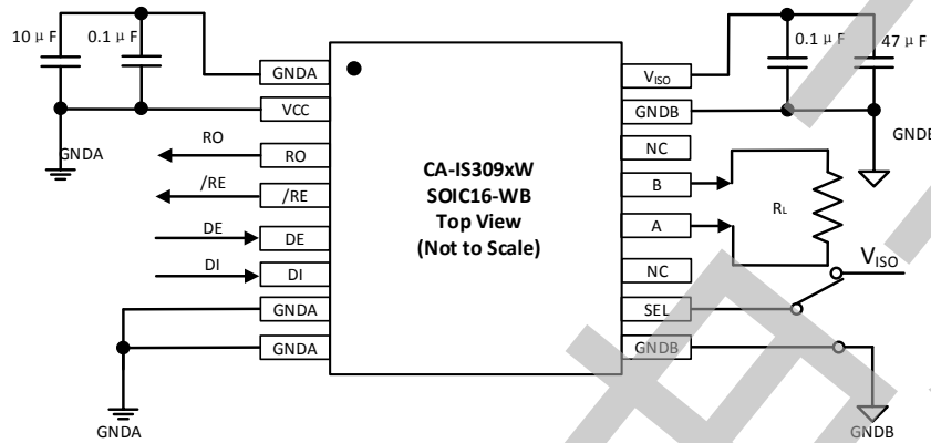
图 12-1 CA-IS309xW 典型应用电路
