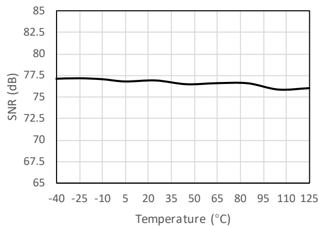
图 7-9 信噪比 vs 温度 @ f_{IN} = 1 kHz
