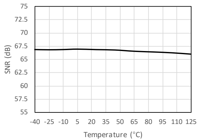
图 7-11 信噪比 vs 温度 @ f_{IN} = 10 kHz
