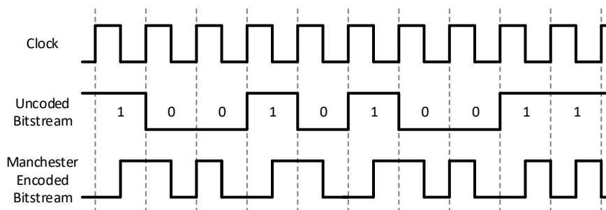
图 8-5 CA-IS1306Ex 曼彻斯特编码的位流波形
