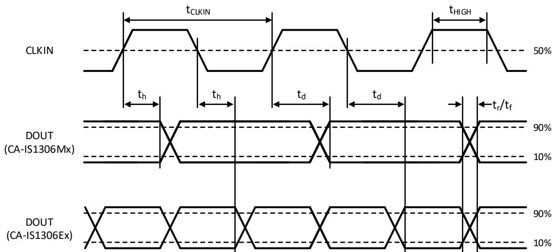
图 7-1 CA-IS1306x 数字输出时序
