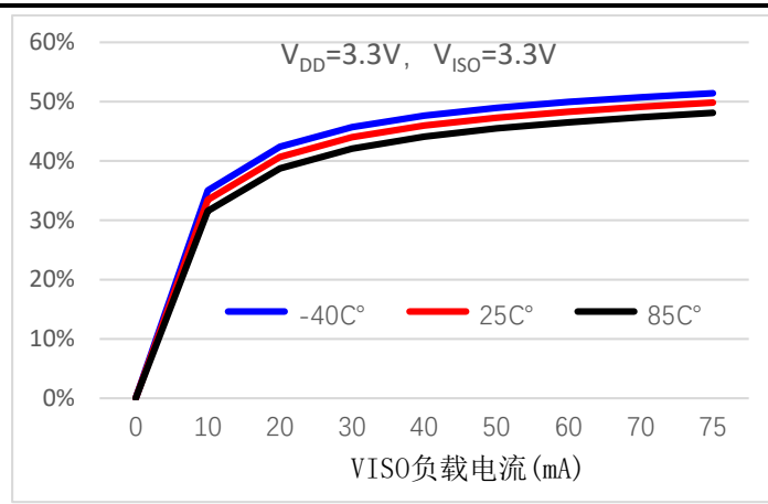
图 8.11-25 不同温度下的效率随器件负载电流的变化 V_{DD} = 3.3V , V_{ISO} = 3.3V
