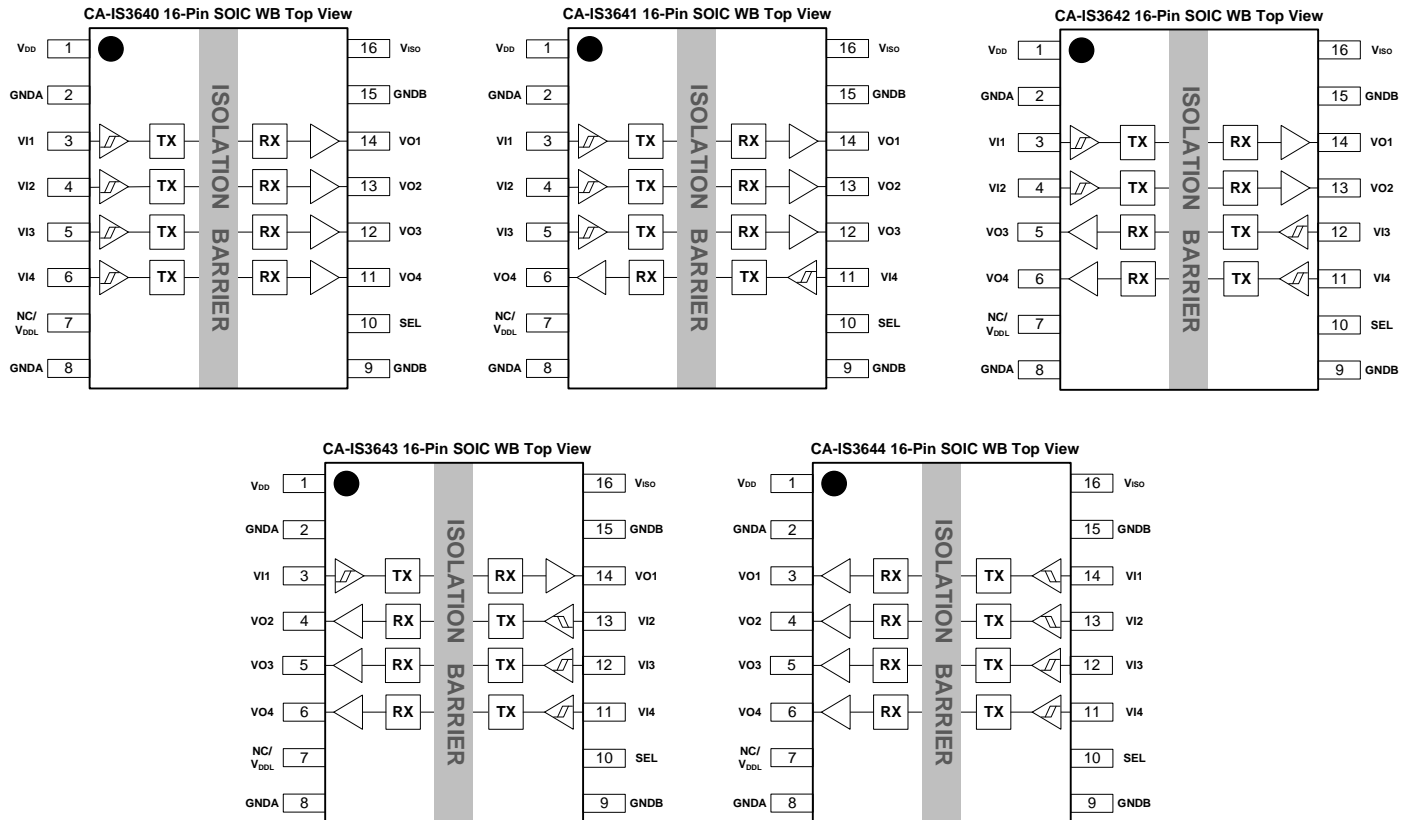
图 7-2 CA-IS364x 顶部视图
