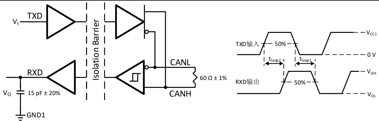
图 8-7 TXD --- RXD 环路延时
