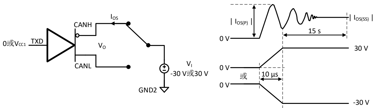
图 8-9 输出短路电流测量电路和波形
