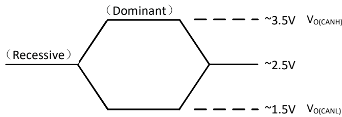
图 8-2 总线逻辑状态的电压定义
