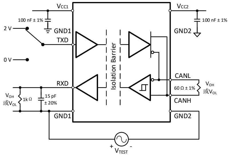
图 8-10 共模瞬态抑制(CMTI)测量电路
