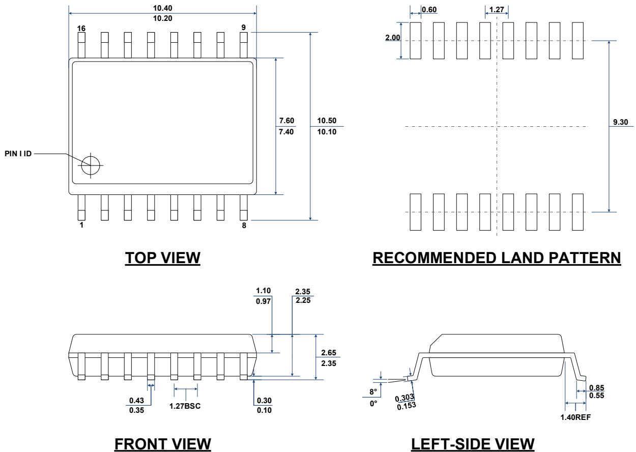
图 11-3 SOIC16-WB 外形尺寸
