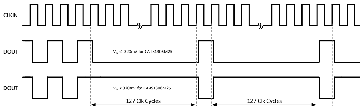
图 8-7 CA-IS1306x 超量程输出波形
