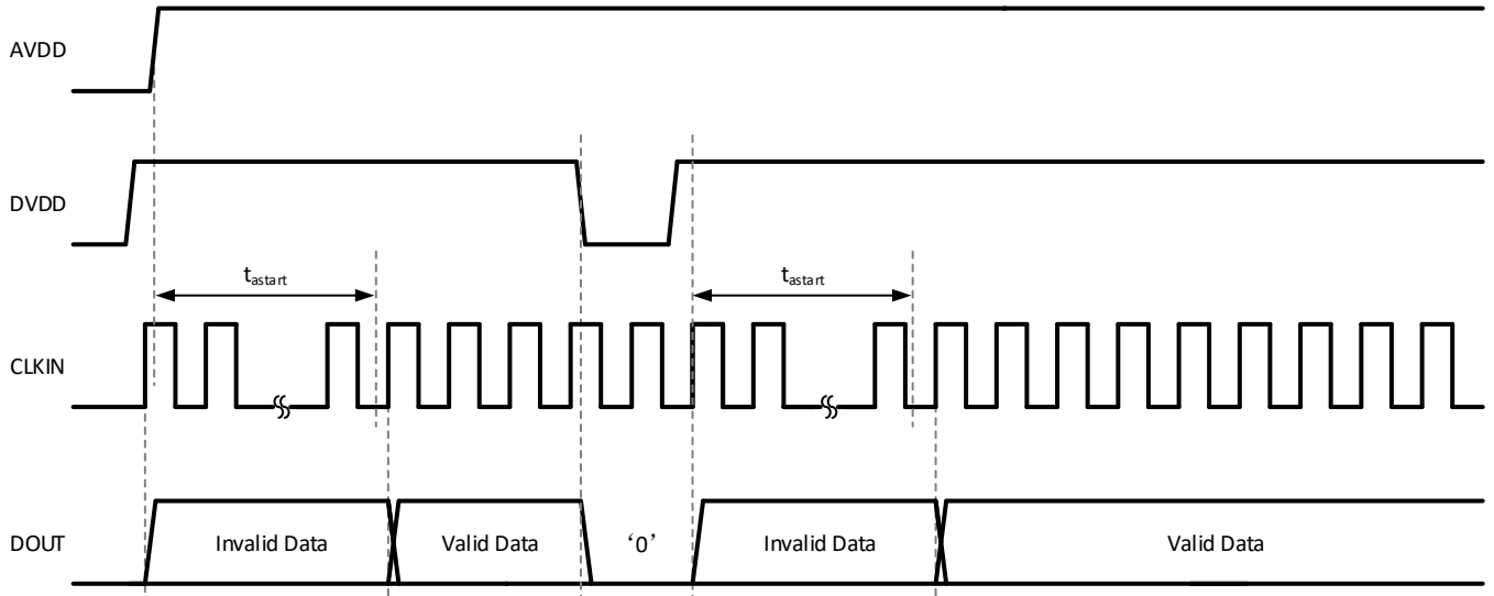
图 7-2 CA-IS1306x 启动时序
