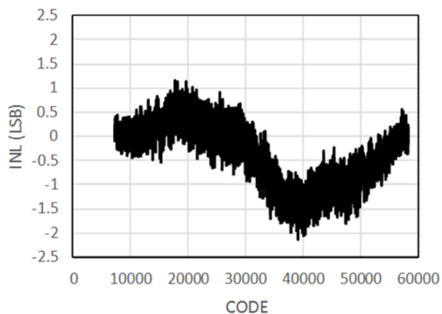
图 7-29 典型积分非线性
