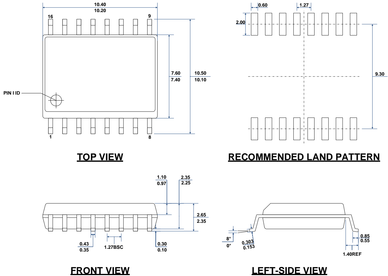
图 10-2 SOIC16 宽体封装外形尺寸图
