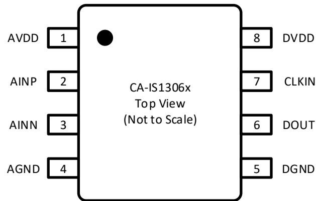
图 6-1 CA-IS1306x 引脚配置
