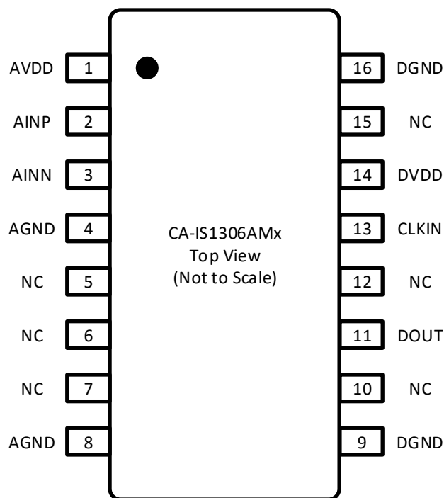
图 6-2 CA-IS1306AMx 引脚配置
