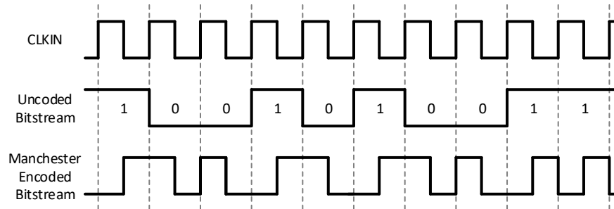
图 8-5 CA-IS1306Ex 曼彻斯特编码的位流波形
