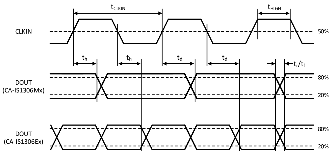
图 7-1 CA-IS1306x 数字输出时序
