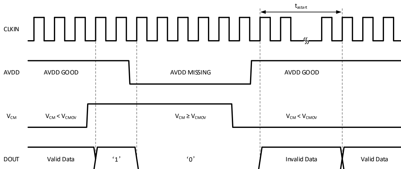
图 8-6 CA-IS1306x 安全故障输出波形
