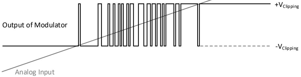
图 8-4 CA-IS1306x 调制器输出与模拟输入 (A1NP - A1NN) 的关系
