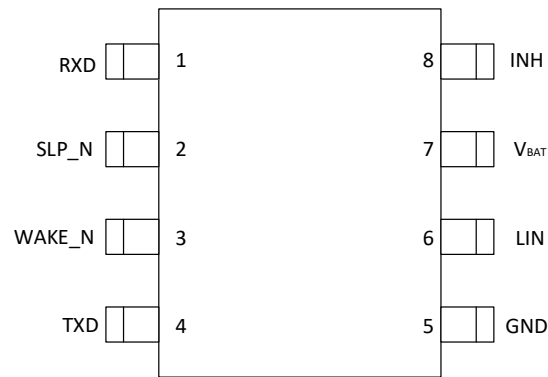
图 6-1 CA-IF1021 引脚图
