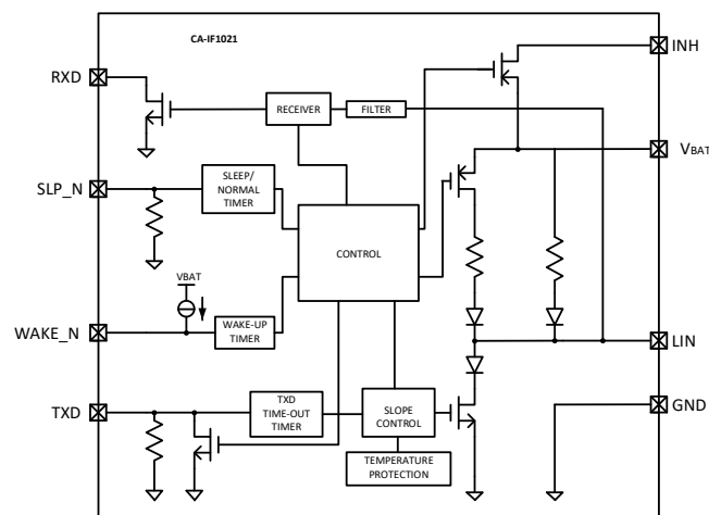
图 3-1 简化芯片结构图
