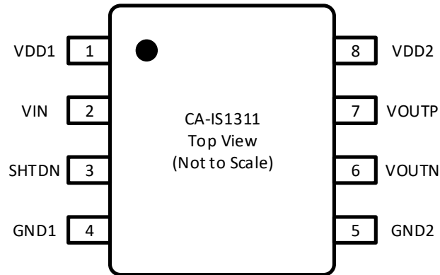
图 6-1 CA-IS1311 引脚配置
