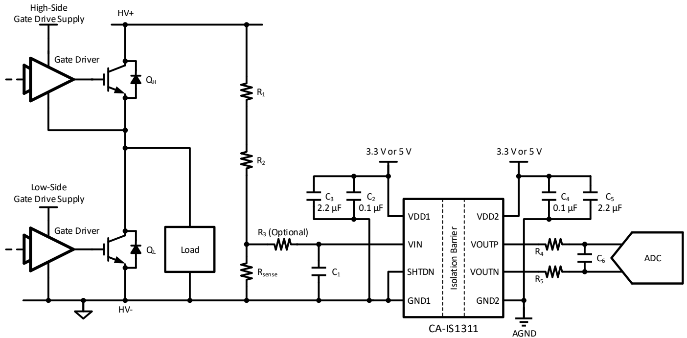
图 10-1 电压检测的典型应用
