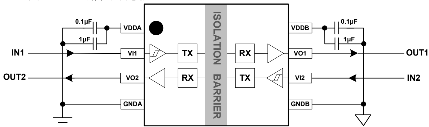
图 10-1 CA-IS3721Cx 典型应用电路
