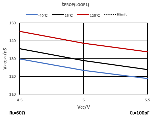
图 8-20 Loop Delay
