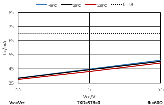
图 8-4 60Ω 负载下显性状态电流
