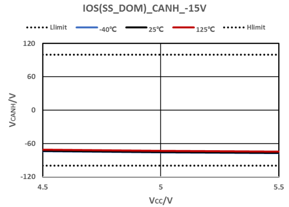
图 8-19 总线短路电流
