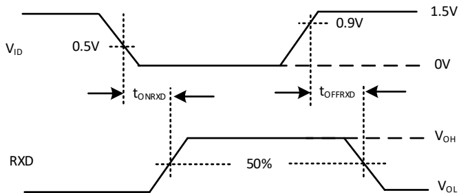
图 7-2 RXD 延迟示意图
