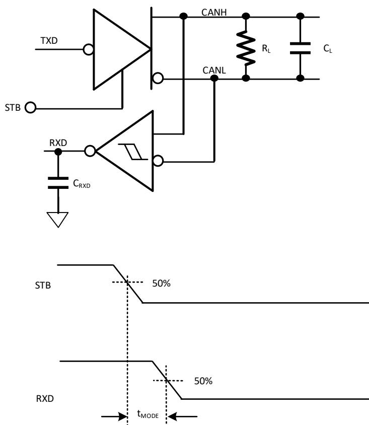
图 7-4 待机态到常态响应示意图
