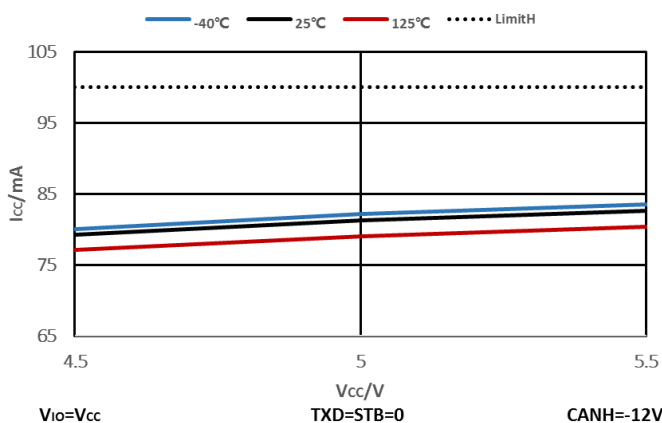
图 8-5 BusFault 电流
