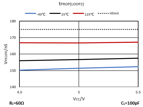
图 8-21 Loop Delay
