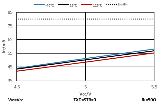
图 8-3 50Ω 负载下显性状态电流
