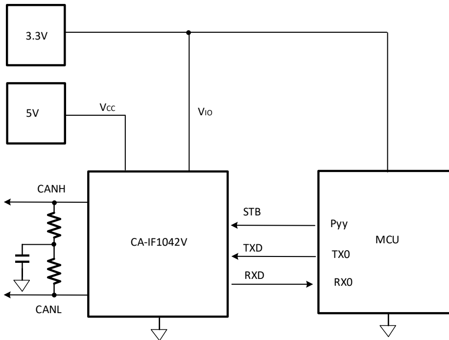
图 10-2 CA-IF1042V CAN 总线典型应用图
