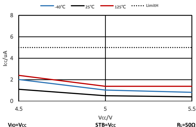
图 8-1 静默态电源电流
