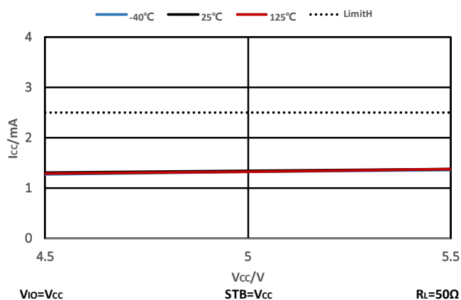
图 8-2 隐性状态电流
