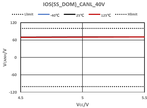
图 8-18 总线短路电流
