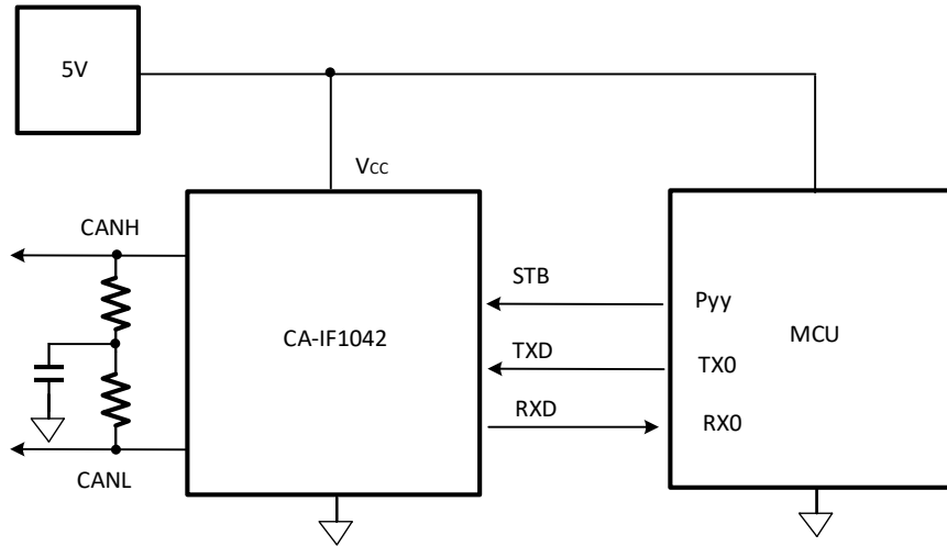
图 10-1 CA-IF1042 CAN 总线典型应用图
