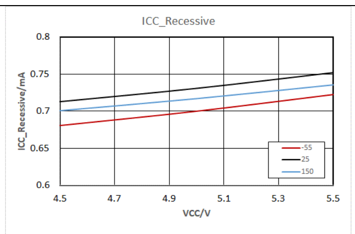
图 9-2 隐性状态电流
