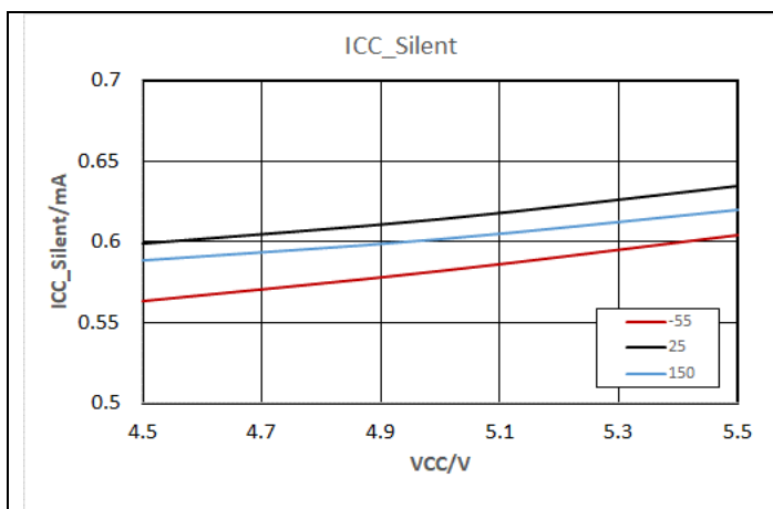
图 9-1 静默态电流
