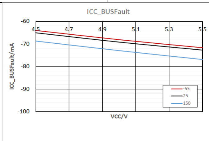
图 9-5 BusFault 电流
