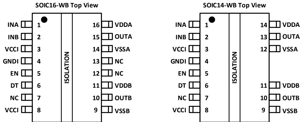
图 6-2. CA-IS3222 引脚配置(SOIC16/SOIC14 封装)
