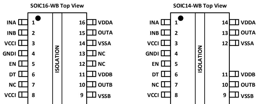
图 6-2. CA-IS3222-Q1 引脚配置(SOIC16/SOIC14 封装)
