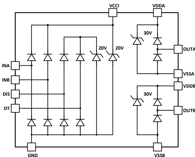
图 9-4. ESD 保护电路
