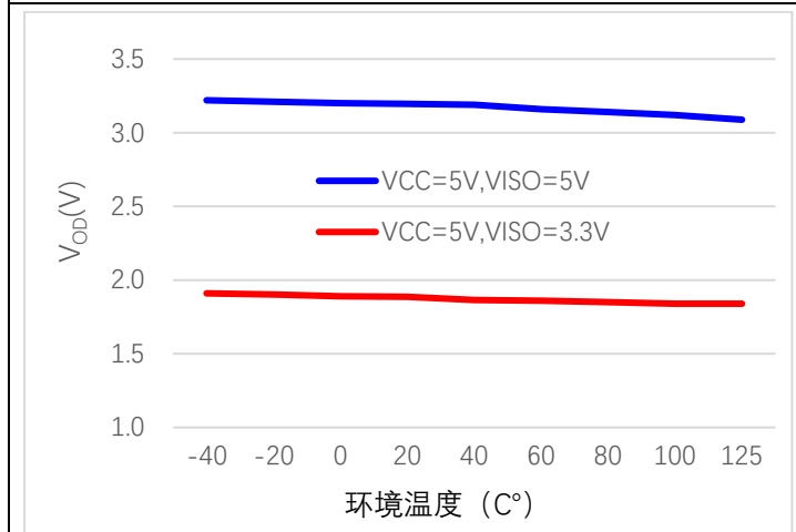
图 7.10-11 差模输出电压 V_{OD} , R_L = 54\Omega , V_{CC} = 5V
