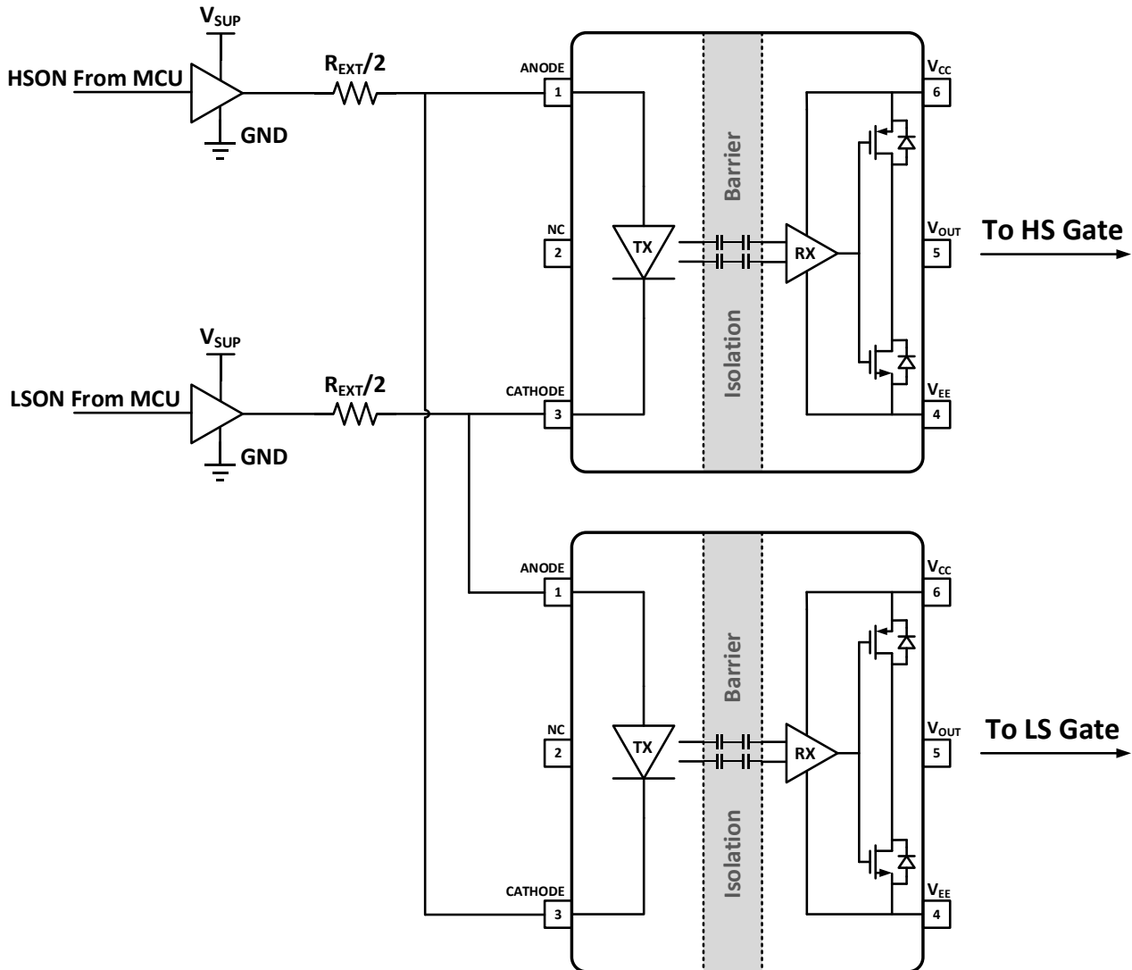
图 10-3 互锁配置
