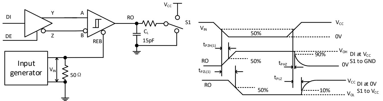
图 7-7 在使能驱动器的情况下测量接收器启用/禁用时间
