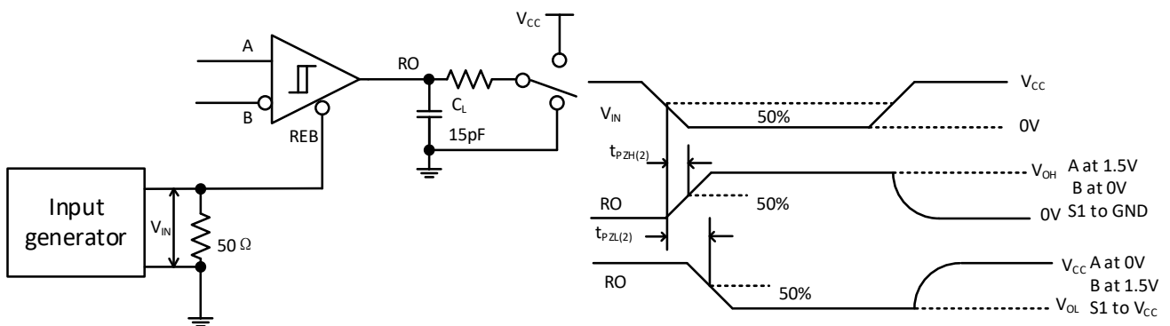
图 7-8 在禁用驱动器的情况下测量接收器使能时间
