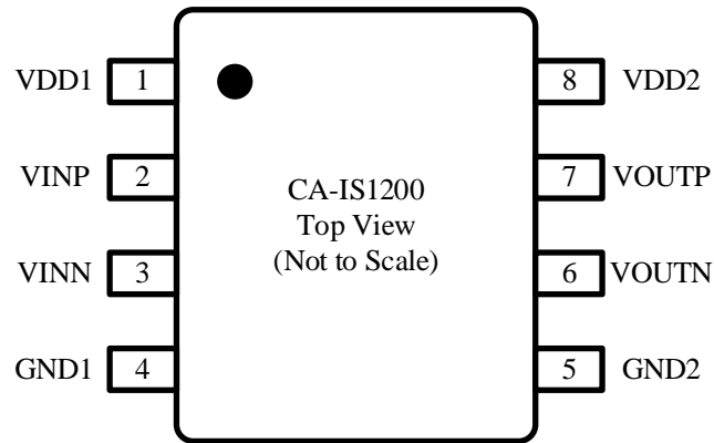
图 6-1 CA-IS1200 引脚配置
