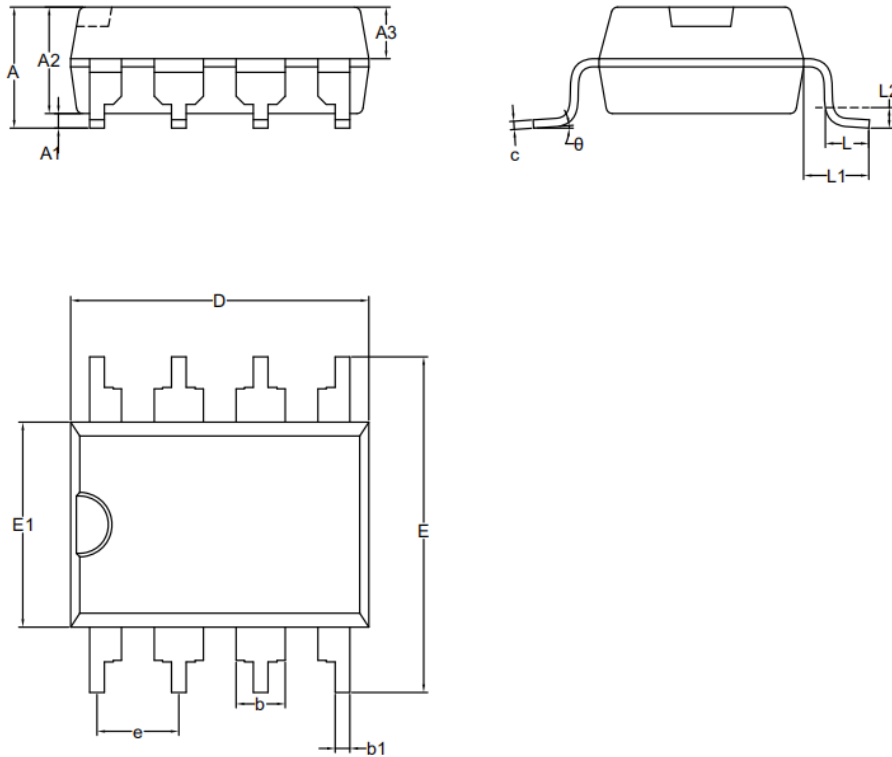
图 11-1 DUB8 封装外形尺寸图
