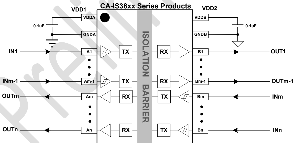
图 9-2 CA-IS38xx 系列数字隔离器应用原理图
