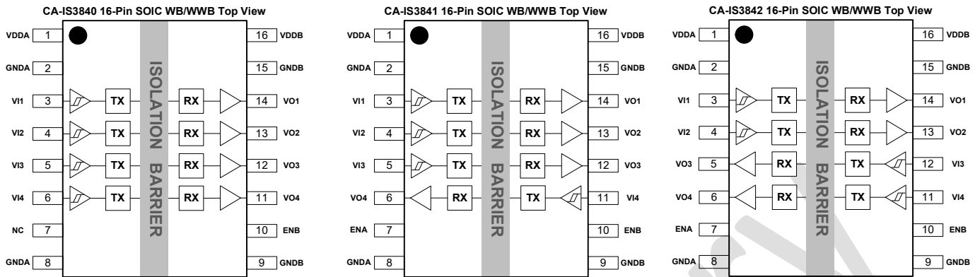
图 5-1 CA-IS384x 顶部视图
