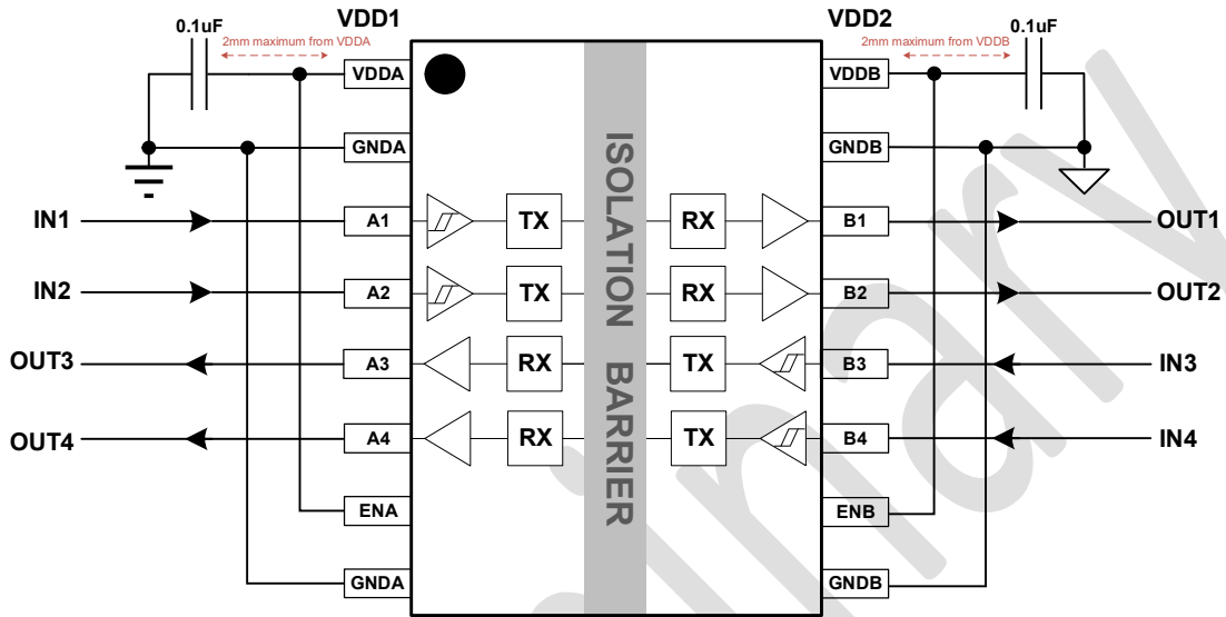
图 9-1 CA-IS3842 典型应用电路
