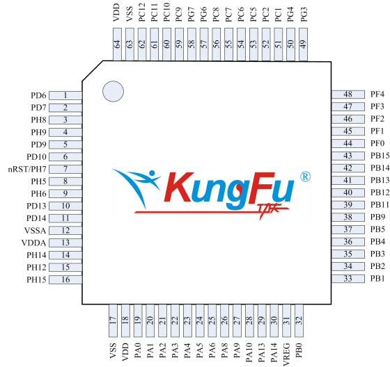
图 2-2 LQFP64
