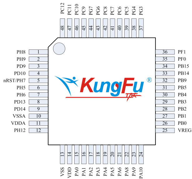
图 2-3 LQFP48
