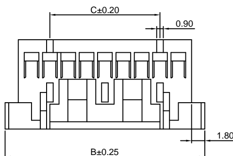
2x9P~2x20P
