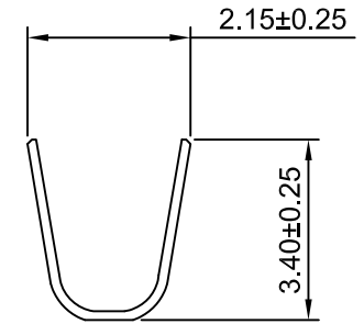
SEC:A-A
