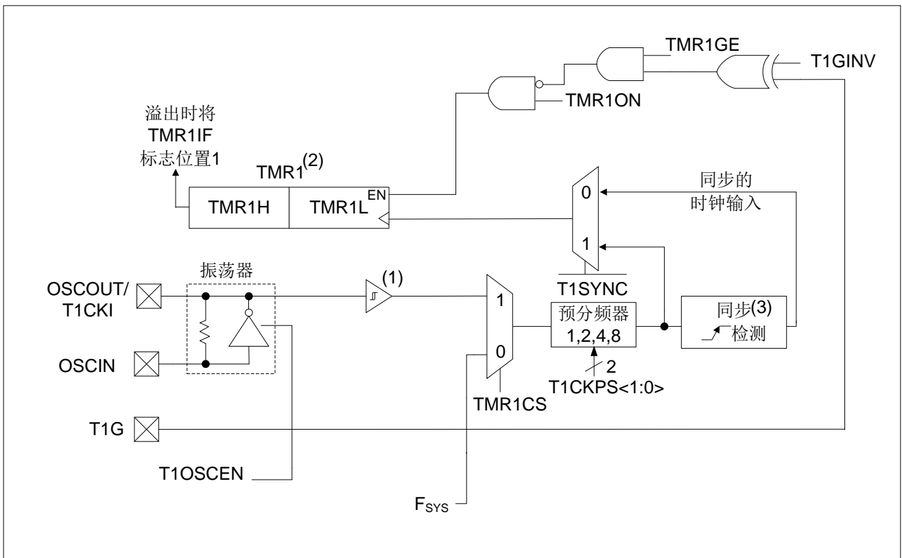
图9-1: TIMER1结构图
