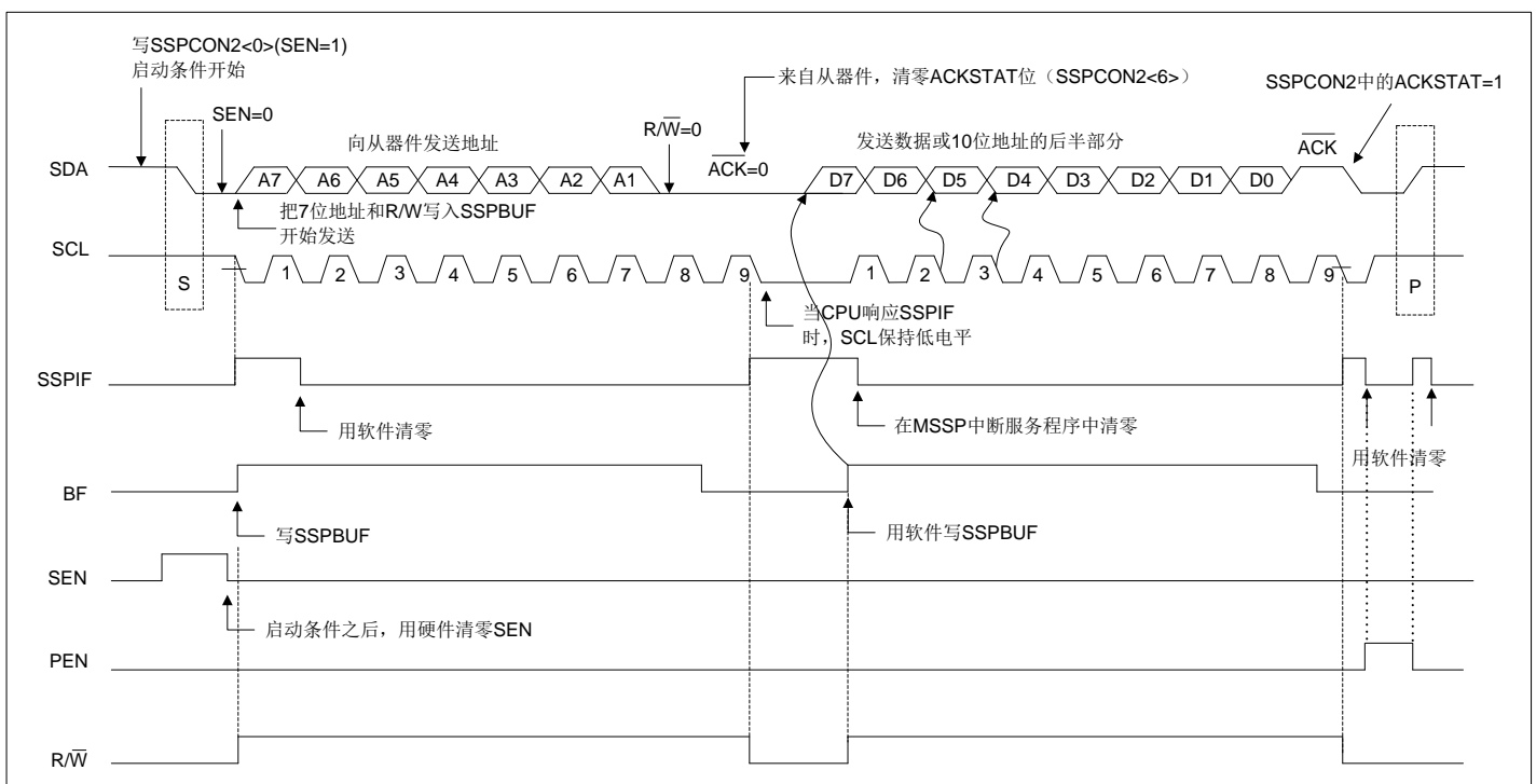
图15-10: I 2 C™主控模式发送时序 (7位或者10位地址)
