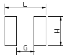
Land Pattern (Unit:mm)
