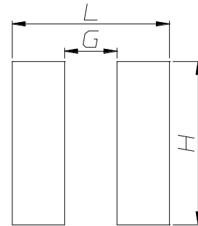
Land Pattern (Unit:mm)
